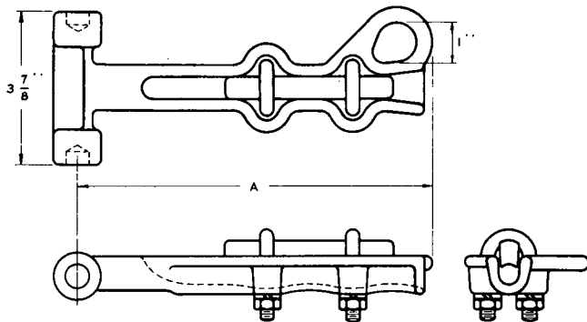
Slack Span Clamp
